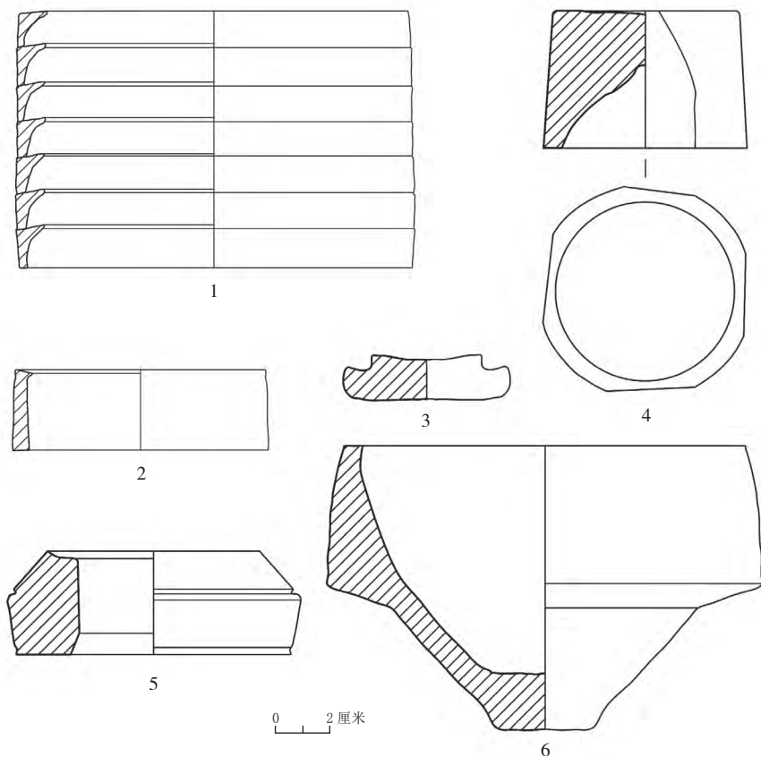
1. 支圈(安后山采:10) 2. 荡箍(安后山采:11) 3. 垫饼(马坪采:18) 4. 轴顶碗(马坪采:8) 5. 匣钵(马坪采:17) 6. 匣钵(碗厂采:13)
