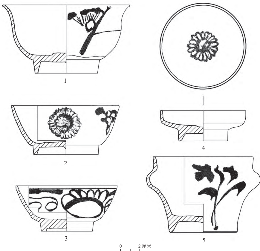
1. 侈口碗(碗厂采: 11) 2、3. 敞口碗(碗厂采: 10、碗厂采: 12) 4. 碟(碗厂采: 8) 5. 罐(碗厂采: 9)
